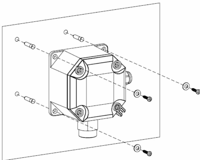
Рис.4 Крепление сенсора
